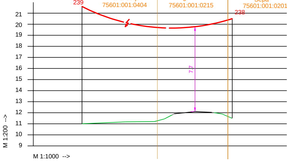
Ristmevälja joonis RV-2
