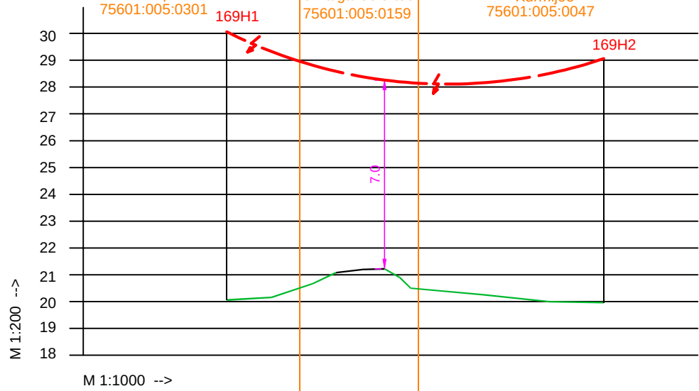
Ristmevälja joonis RV-4
