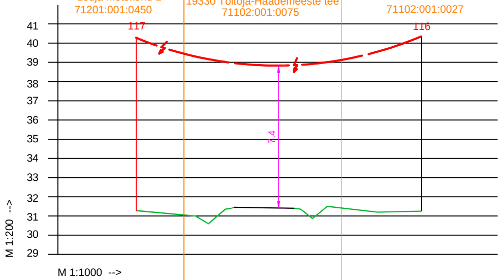
Ristmevälja joonis RV-5
