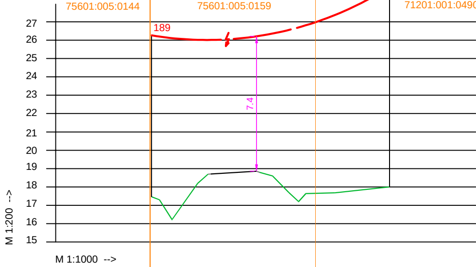
Ristmevälja joonis RV-3
